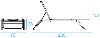
504 Lettino impilabile Stackable sunbed W200 - D75 - H38/101 Kg 15,4
