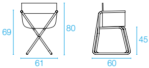
213 Poltroncina regista Director's armchair W61 - D60 - H80 Kg 7,8
