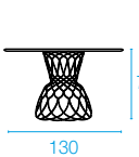
570B+570P Tavolo tondo 6 posti 6 seats round table ø130 - H74 Kg 29,2
