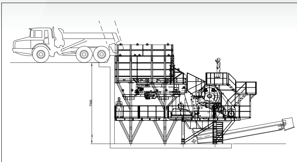
Schematisk bild över hela krossanläggningen som den ska se ut med den nya förkrossen och övrig anpassning
