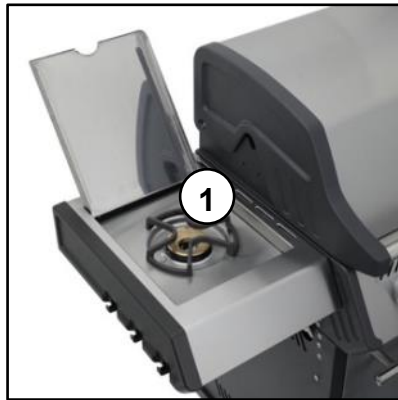
Abb. 20 - Seitenkocher
