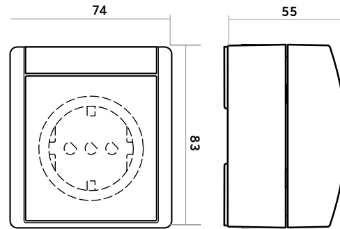
Steckdose 1-fach
