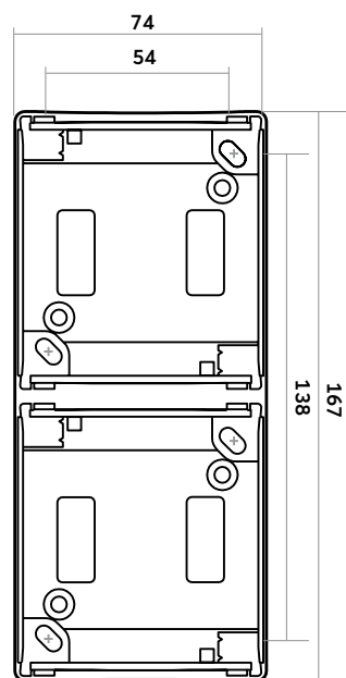
AP-Dose 2-fach senkrecht
