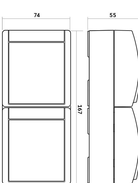
Schalter 2-fach senkrecht
