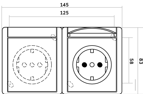
Steckdose 2-fach waagerecht
