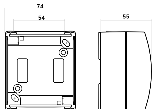
AP-Dose 1-fach waagerecht
