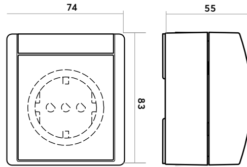
Steckdose 1-fach
