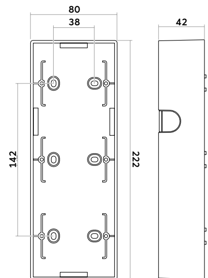
AP-Gehäuse 3-fach
